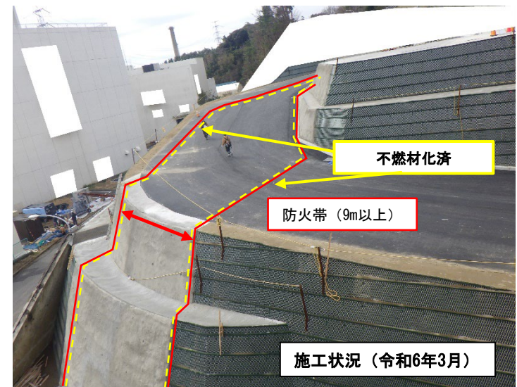
防火帯設置場所の施工状況
